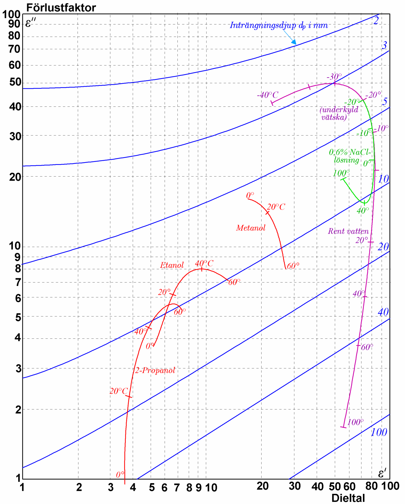
Permittivetsdiagram vid 2450 MHz med d_p som parameter
